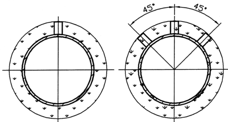
Схема установки скобы опорной.
