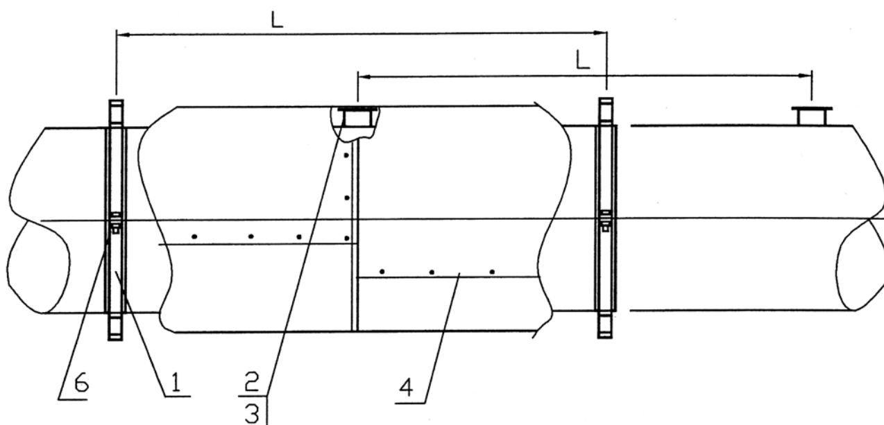
Схема установки скобы опорной.
